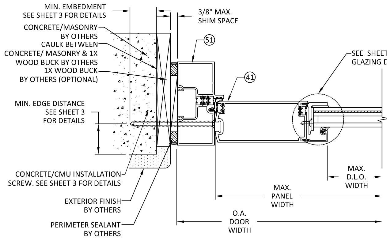
A HORIZONTAL SECTION 6 500T DOOR & TRIFAB 451T SUBFRAME JAMB-CONCRETE/CMU
